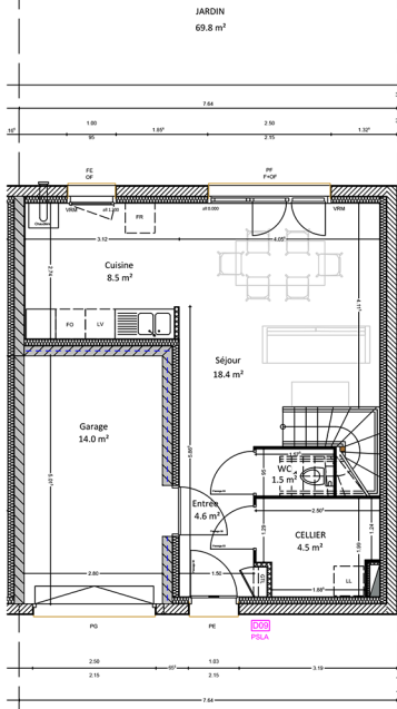
PLAN RDC
